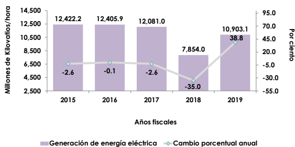
Gráfica 31 GENERACION DE ENERGÍA ELÉCTRICA PUERTO RICO, PERÍODO DE JULIO - ENERO AÑOS FISCALES 2015 - 2019
